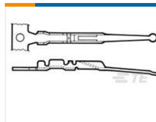
TE 产品编号 66555-2 TYPE CR ACTIVE CONTACT
