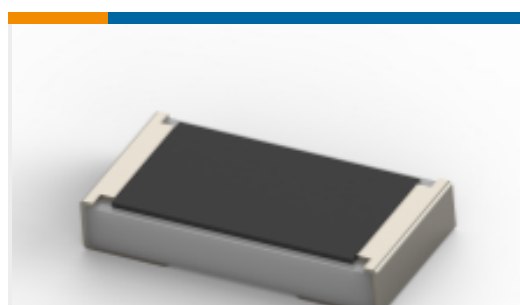
TE 产品编号2176232-4 SMD 功率电阻器: 3 瓦特, 1% Tol
