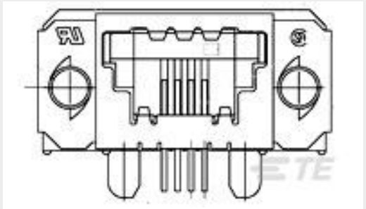
TE 产品编号5-1761185-1 4 SDL SE GRND RCPT ASSY
