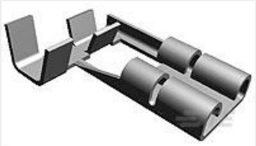
TE 产品编号100645-3 250 FASTON,FLAG,REC.,14-17AWG, PHBRZ
