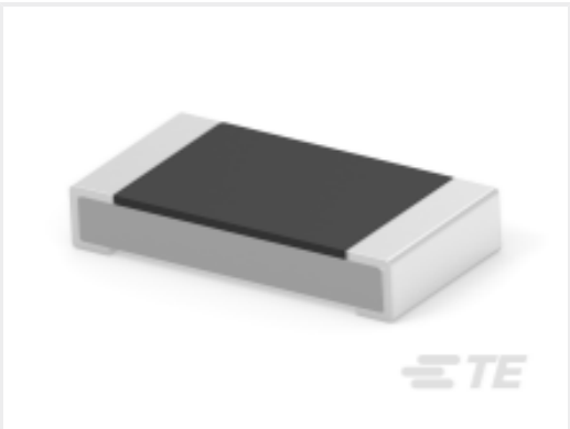
TE 产品编号7-2176392-0 RQ 1206 698K 0.1% 10PPM 5K RL
