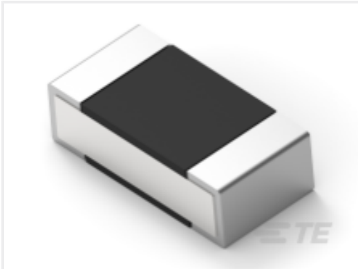
TE 产品编号1-2176305-1 RP 1E 0.1W 137R 0.1% 25PPM 5K RL
