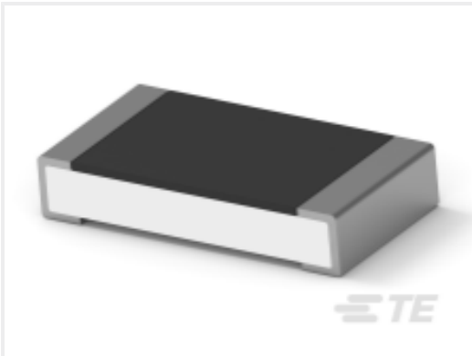
TE 产品编号1-2176391-5 RQ 1206 17K4 0.1% 10PPM 5K RL
