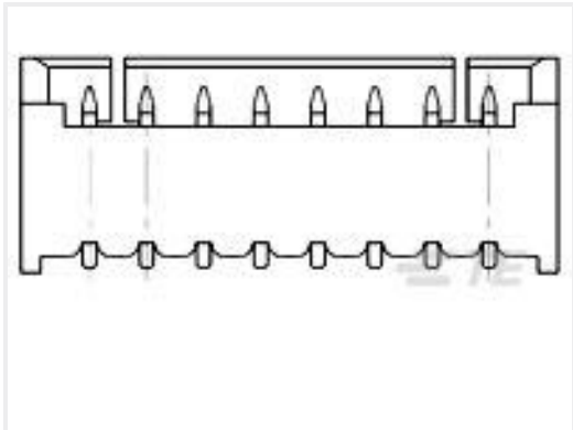
TE 产品编号1734829-8 1.25 WTB HDR DIP, 8 POS
