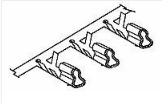
TE 产品编号440134-1 2.5mm,Crimp Contact
