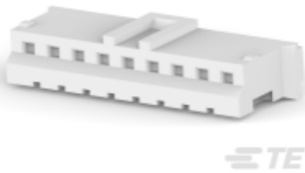
TE 产品编号 440129-9 2.0MM,HSG,9POS
