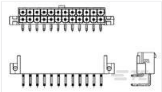
TE 产品编号1586044-6 6P VAL-U-LOK R/A HDR SCR MT V0
