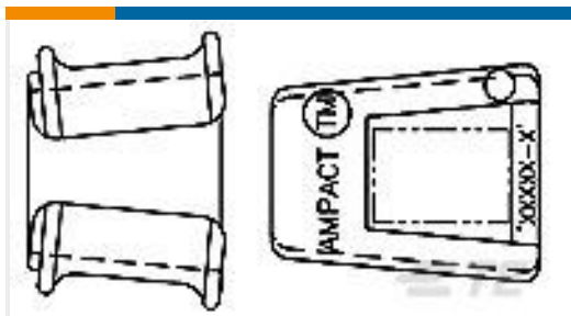
TE 产品编号1974127-1 铜质剪切螺栓接头，适应高达 35 kV 的电压
