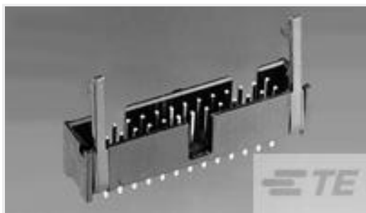
TE 产品编号104130-5 026 LOPRO HDR RA 30DP LATCH
