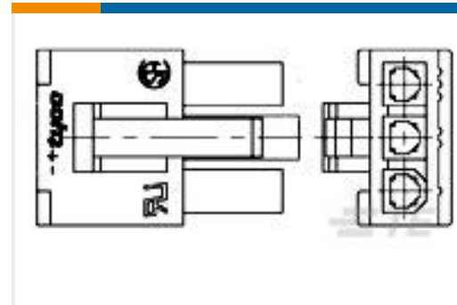
TE 产品编号2029112-3 3P RCPT SR VAL-U-LOK GW
