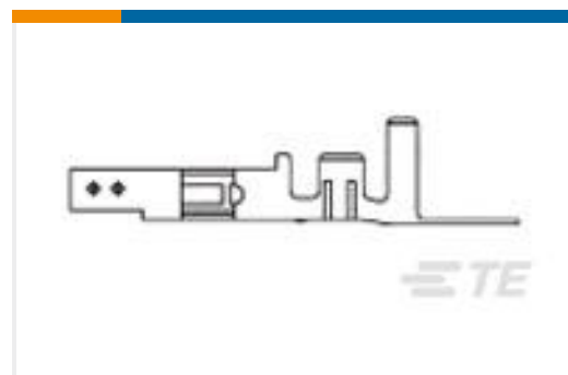
TE 产品编号2238017-1 VAL-U-LOK SKT BR SN 18-22AWG
