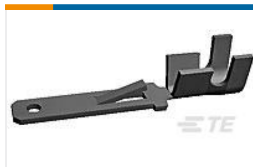
TE 产品编号60294-1 FF 250 TAB 22-18AWG BR
