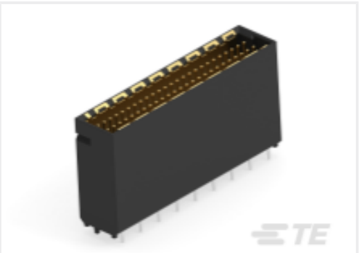
TE 产品编号224562-E MSPEED 50 M SMDTHR M10 * AB VV 137 176 *
