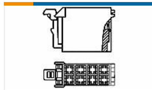
TE 产品编号144172-2 MODULE 8 POS ASSY
