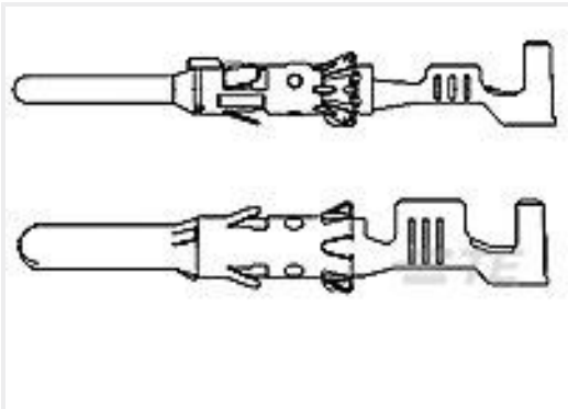
TE 产品编号929962-1 STIFTKONTAKT 2,5MMD
