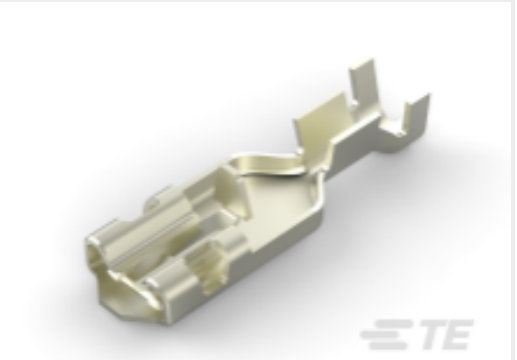
TE 产品编号2238104-1 250 PL MKII REC. 16-14AWG NPST
