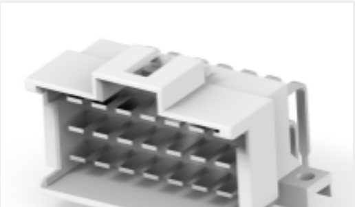
TE 产品编号8-966140-6 TAB HEADER 2.8 X 0.8 MM 21 POS
