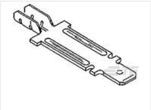
TE 产品编号63301-1 250 FASTON TAB 22-15 AWG NPST
