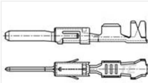
TE 产品编号963900-1 TAB A 1.6x0.6 CONTACT CS SRC Sn
