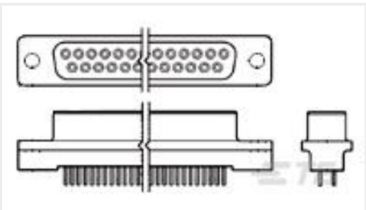
TE 产品编号5207826-4 HD-20 RCPT 9P VERT
