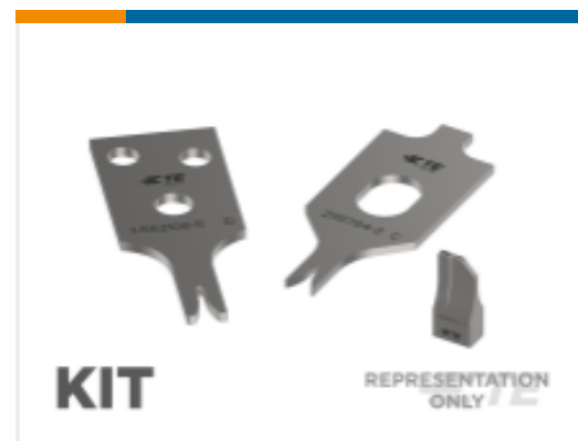
TE 产品编号 7-2151911-7 OC-080F1600-752- CRIMPTOOLINGKIT
