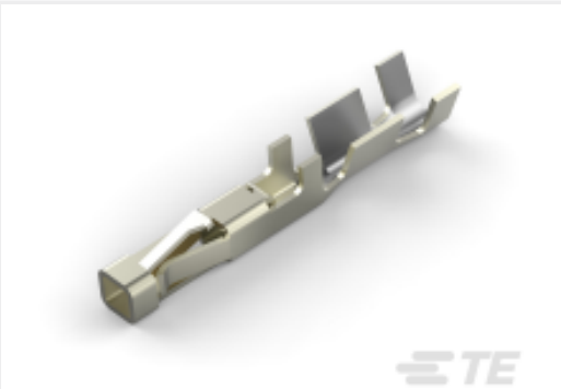
TE 产品编号1-794606-3 MICRO MNL RPT CNT STRP 30AU LF
