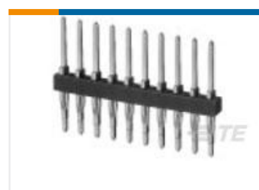
TE 产品编号8-102898-3 40 MODII HDR SRST UNSHRD A/PIN
