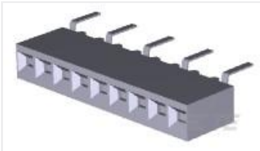
TE 产品编号5-147727-8 09 MODIV VRT SR OUTRIGGER SN
