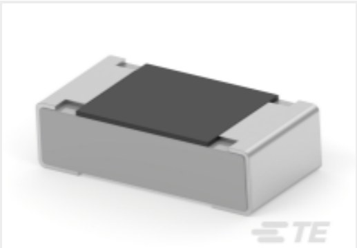
TE 产品编号4-2176340-3 CRGCQ 0603 10M 5%
