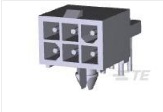
TE 产品编号1-770969-1 06P MINI UMNL R/A HDR ASSY LF
