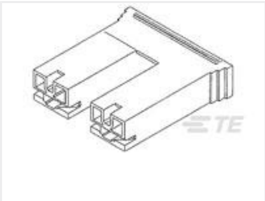
TE 产品编号1-520935-1 250 HSG. PL MKII REC. 15.11mm 2P NAT
