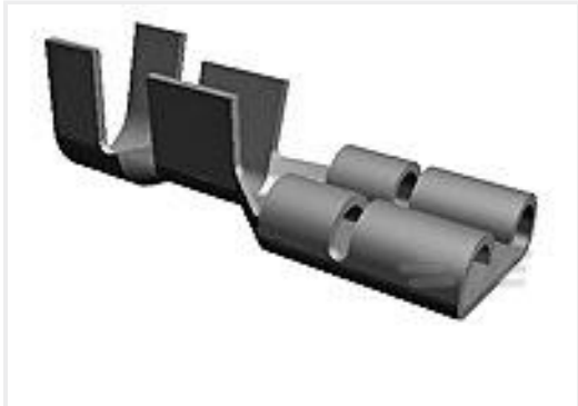
TE 产品编号63674-1 250 FASTON REC 18-14 AWG NPST
