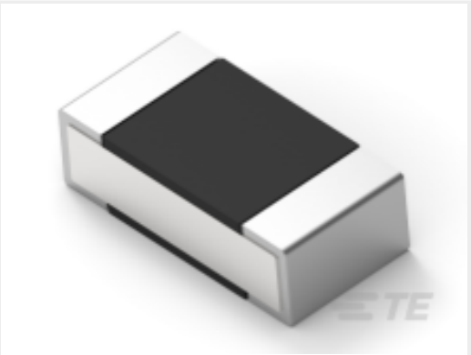
TE 产品编号4-2176307-3 RP 1E 0.1W 34K 0.1% 25PPM 5K RL
