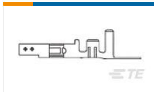
TE 产品编号794956-1 VAL-U-LOK SKT BR SN 22-18AWG
