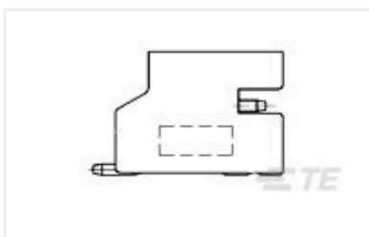
TE 产品编号1-1775469-0 HPI CONN., 2.0MM, R/A, SMT, 10P, 80U"
