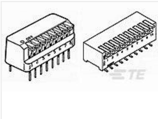
TE 产品编号435802-8 RIGHT ANGLE DIP SW 10 POS AU
