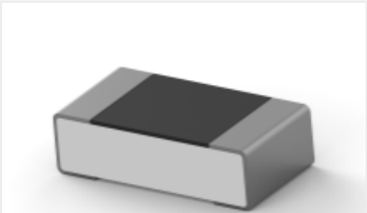
TE 产品编号4-2176369-2 RQ 0603 107R 0.1% 10PPM 5K RL
