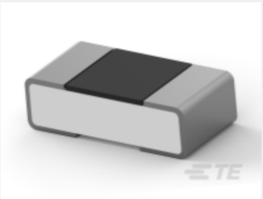
TE 产品编号6-2176364-1 RQ 0402 19K6 0.1% 10PPM 5K RL
