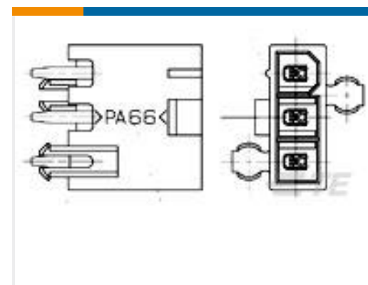
TE 产品编号2029054-4 4P VAL-U-LOK SR HDR SN V2 W/DH
