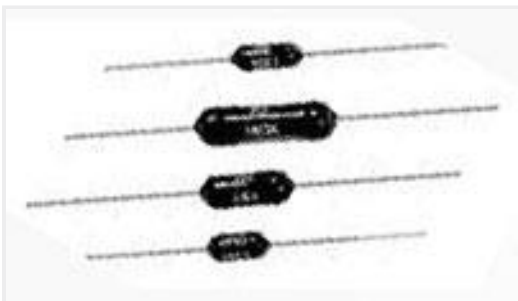
TE 产品编号1-1879665-2 H8 16K2 0.1% 15PPM
