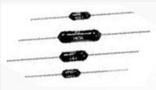
TE 产品编号5-1879619-9 H8 2K7 1% 25PPM
