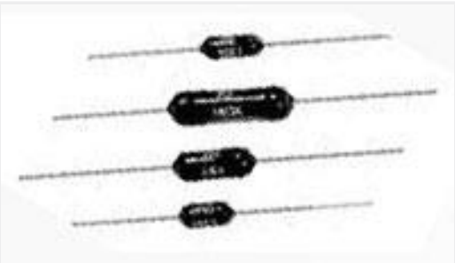
TE 产品编号5-1879642-3 H8 6K0 0.1% 25PPM
