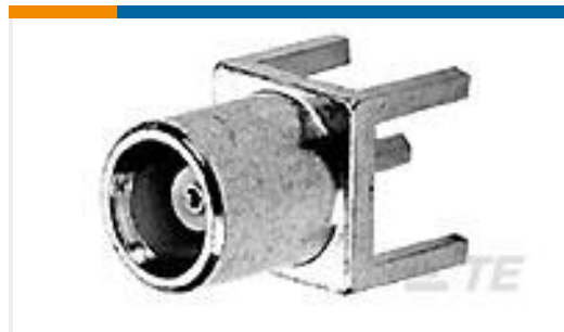
TE 产品编号1-1337581-0 MCX Str PCB Skt 50Ohm Gold Pltd
