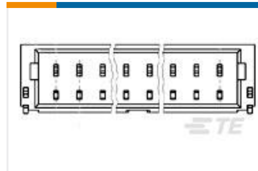
TE 产品编号1-1734709-5 1.0 WTB HDR SR RA 15 POS
