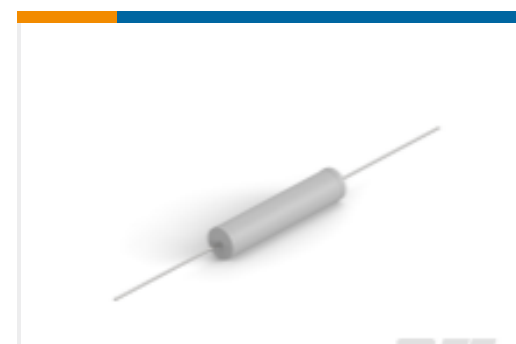
TE 产品编号4-2176415-8 8W STD M/OX 5% 2K7
