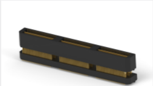
TE 产品编号 2-1658438-3 MSB0.80PL14ASY120FL,-,10,-TY
