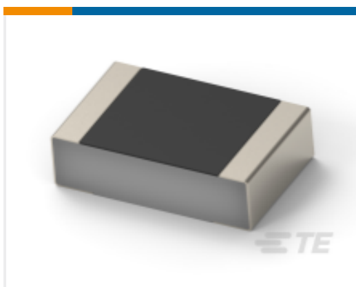
TE 产品编号2-2176453-8 CPF 0201 11K 0.1% 25ppm 1K RL
