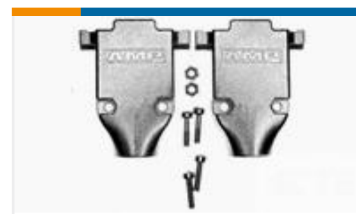
TE 产品编号5748677-4 PLTD PLST CBL CLMP KIT, SZ 4
