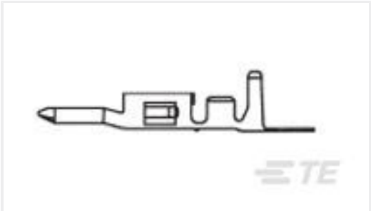
TE 产品编号1586314-2 VAL-U-LOK PIN BR AU 22-18 LP
