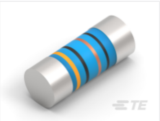
TE 产品编号3-2176316-5 MELF SMA_A 68K 0.1% 15PPM 0207 1W
