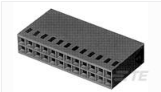
TE 产品编号4-87456-9 04 MODIV HSG COMP DR .100CL
