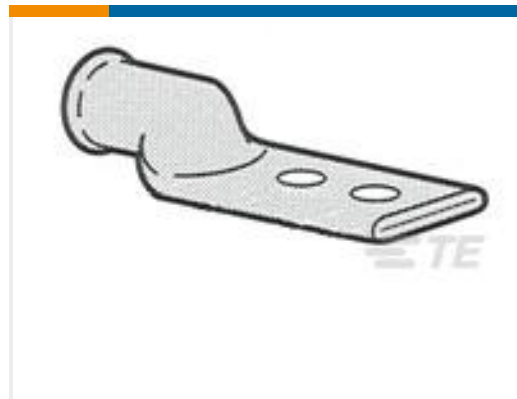
TE 产品编号 53686-2 TERMINAL,AMPOWER 700MCM 1/2
