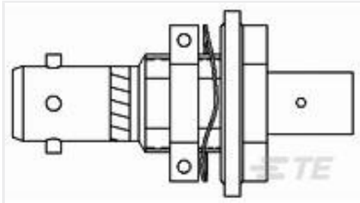
TE 产品编号704201-000 DK-621-0438-3S
