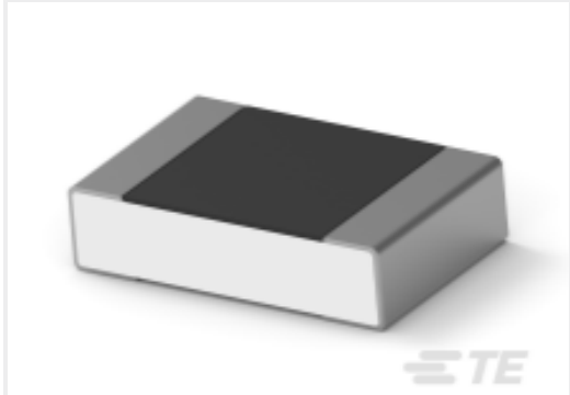
TE 产品编号1-2176381-9 RQ 0805 19K1 0.1% 10PPM 5K RL
