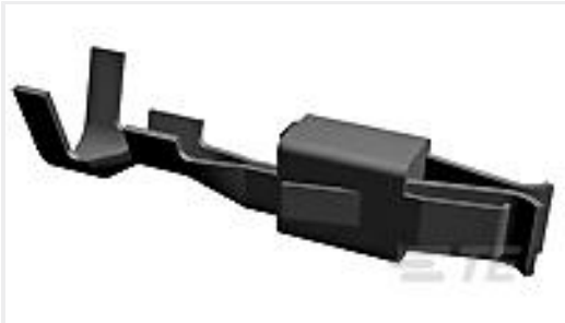
TE 产品编号929941-3 JPT REC 2.8 Contact SWS Sn
