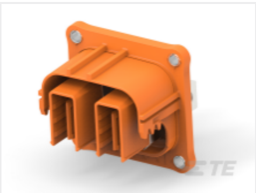
TE 产品编号 3-2344512-1 2POS,21MM,HEADER HSG,ASSY
