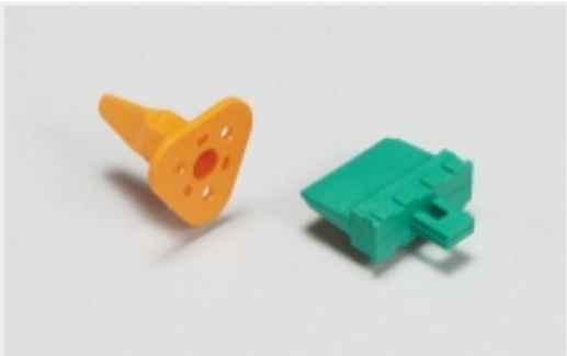
汽车连接器锁和位置保证(3)
