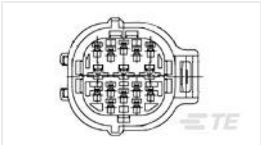
TE 产品编号2-85262-1 E-S MK-2(+) 15P PLUG ASSY
